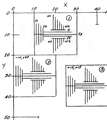
SCREEN COORDINATES
